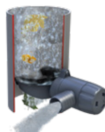
Rapido stuprörsanslutning inkl. håltagare för bormaskin.
